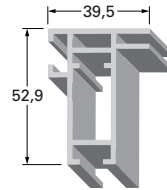
frame 39,5 (System 2) 1,13 kg/m
