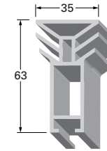
frame 35 D (System 35) 1,45 kg/m
